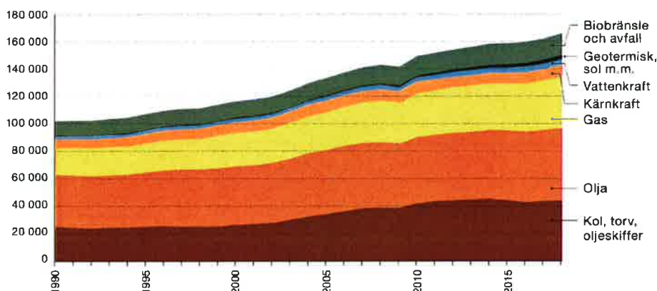
Figur 1. Global tillförsel av energi per energislag. Källa: Energiåret 2021
